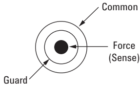
Figure 3.4. SMU terminal
